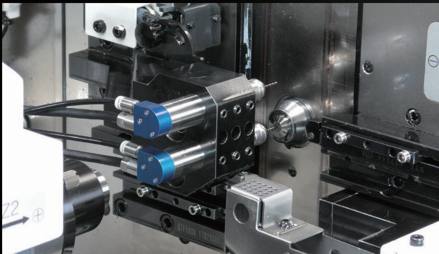
搭載機：シチズンマシナリー株式会社 主軸台移動形 CNC 自動旋盤 Cincom R04
