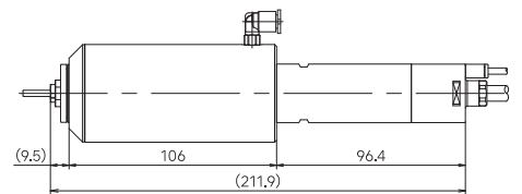
モータ： EM-3060J 接続時寸法
