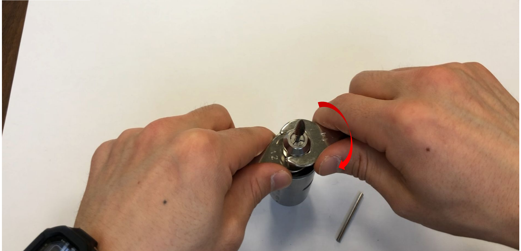
コレットナット及びスピンドル軸を再度スパナで固定し、 時計方向に回して工具を固定
